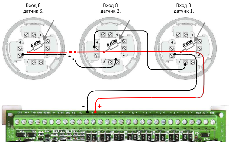
Рисунок 43. Схема подключения пожарных датчиков на вход №8
