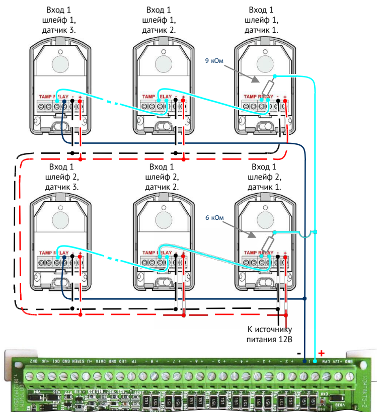
Рисунок 41. Схема подключения охранных датчиков на вход №1
