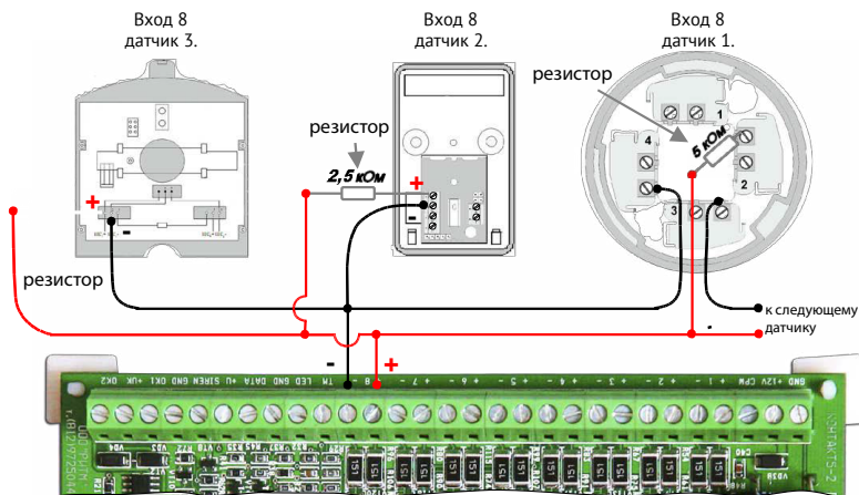
Рисунок 46. Схема подключения пожарных датчиков на вход №8
