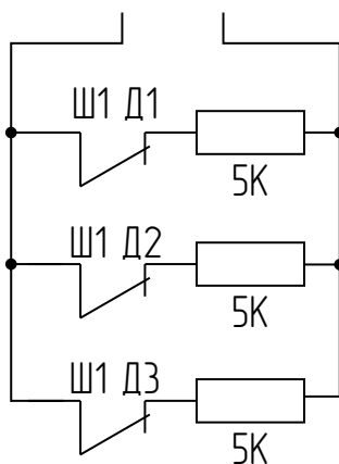
Рисунок 44. Эквивалентная схема для рис. 43
