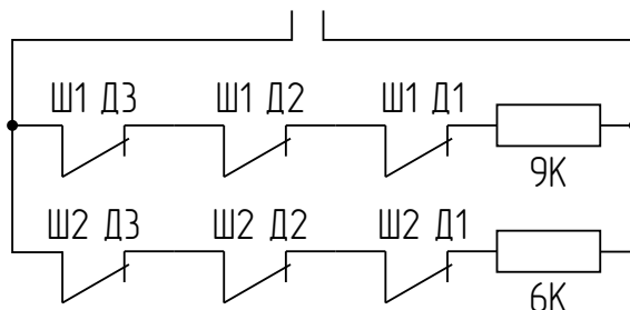
Рисунок 42. Эквивалентная схема для рис. 41
