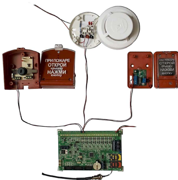
Рисунок 48. Фотография подключения пожарных датчиков
